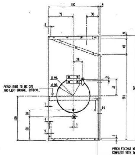
END ELEVATION
