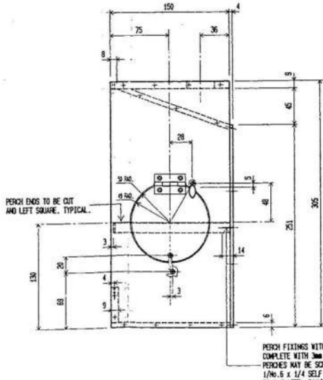
END ELEVATION
